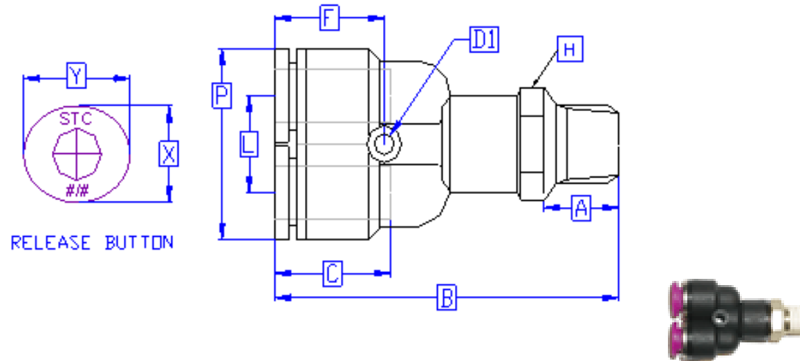
Y Connector
